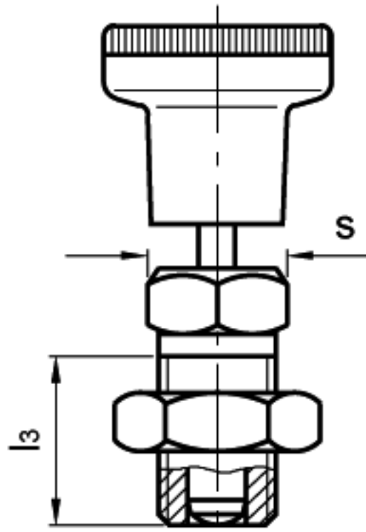
AK 型 (带齿轮脱开锁)
